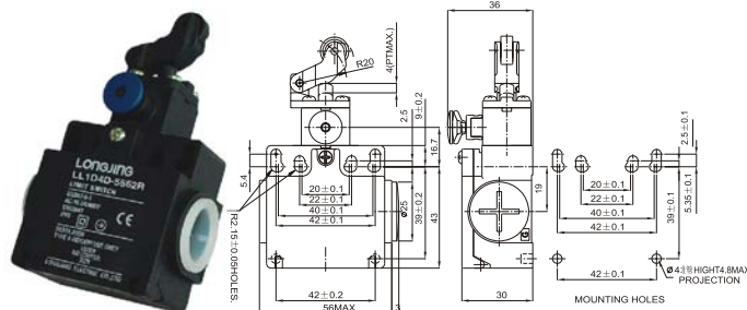
LL1D4D-5562R
