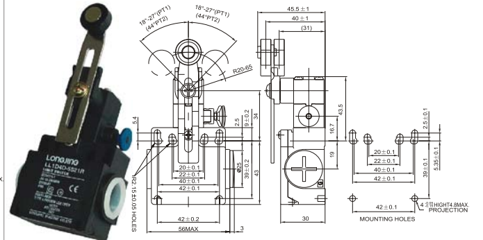
LL1D4D-5521R
