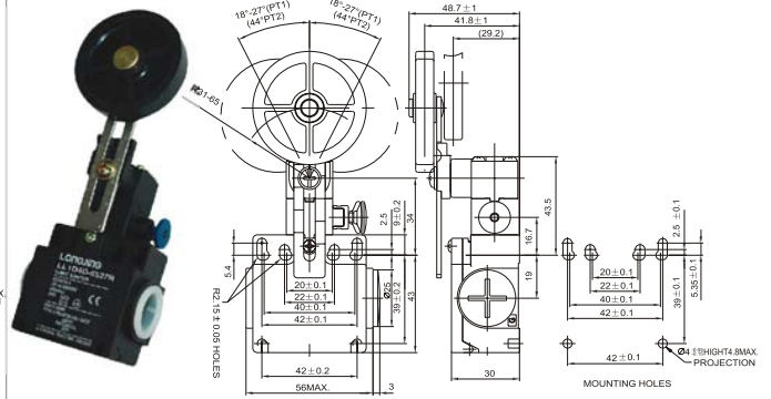
LL1D4D-5527R
