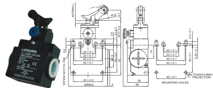
LL1D4D-5572R
