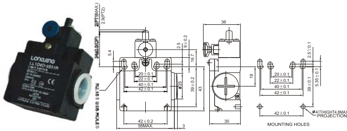
LL1D4D-5531R
