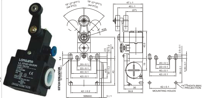
LL1D4D-5520R
